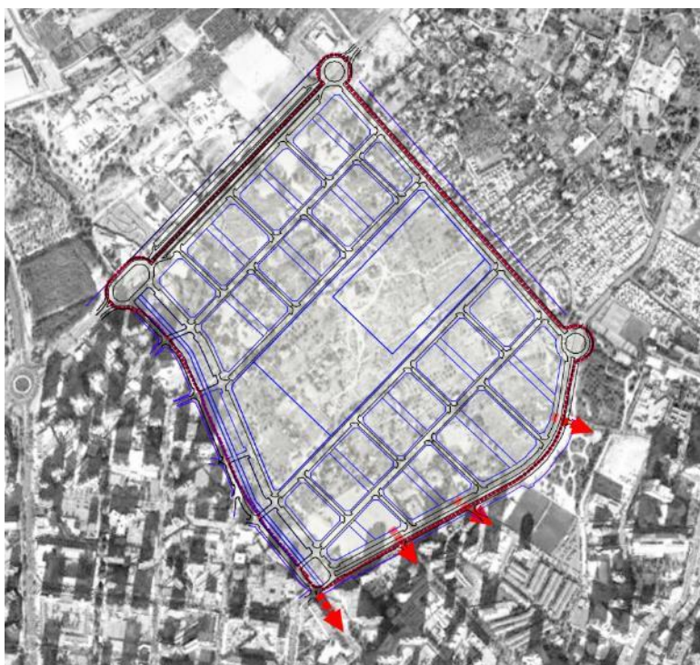
Ilustración 123. Esquema conexiones red de saneamiento de aguas residuales
