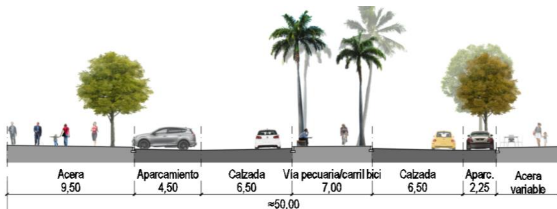
Sección tipo avda. Almirante Bernat de Sarrià
