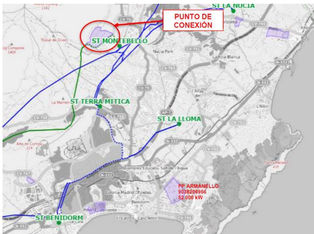
Ilustración 127. Situación punto suministro y trazado infraestructuras de energía eléctrica.
