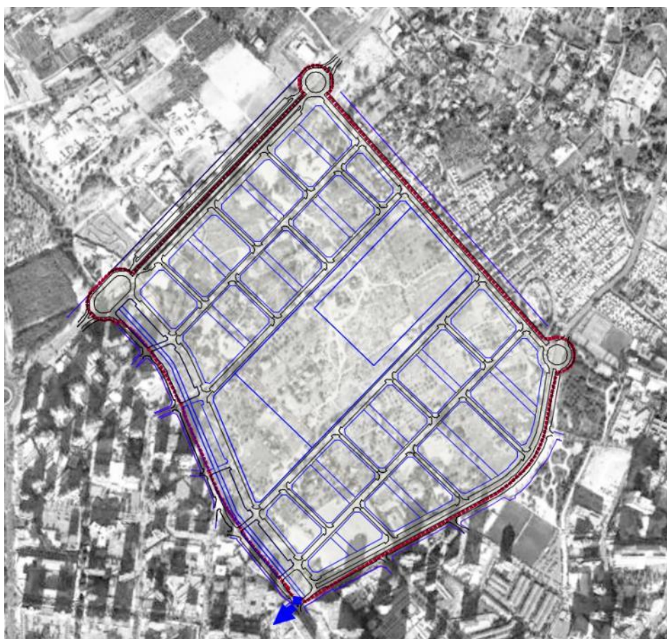
Ilustración 124. Esquema conexiones red de saneamiento de pluviales.
