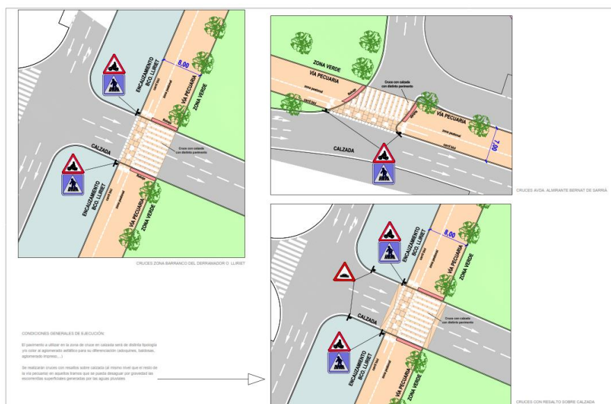
Planta cruce tipo vía pecuaria sobre calzada
